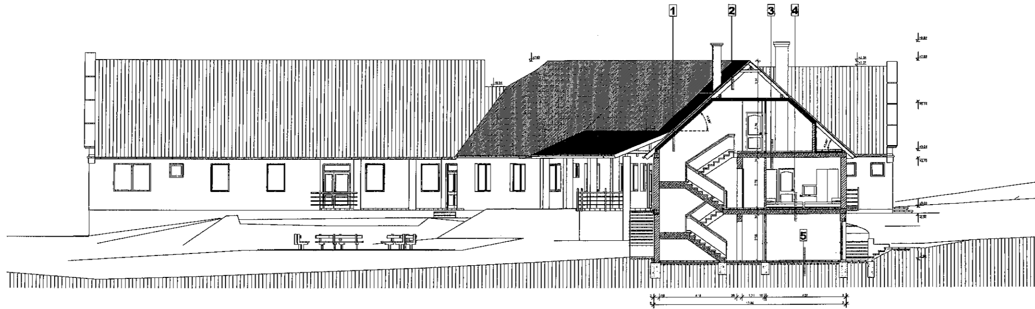
FELMÉRT A-A METSZET M 1:100
